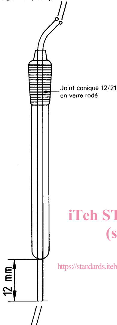
Figure 3 — Électrodes en platine
