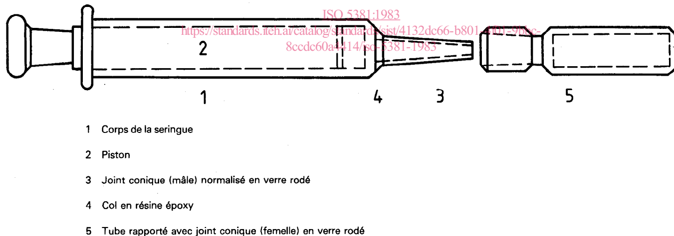
Figure 1 — Seringue spéciale
