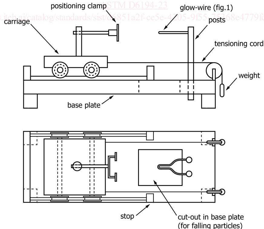
FIG. 2 Test Apparatus (Example)
