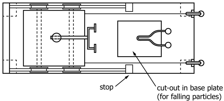
FIG. 2 Test Apparatus (Example)
