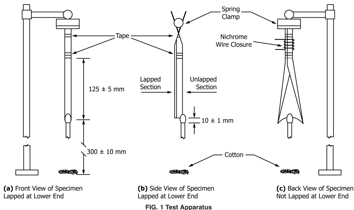
FIG. 1 Test Apparatus
