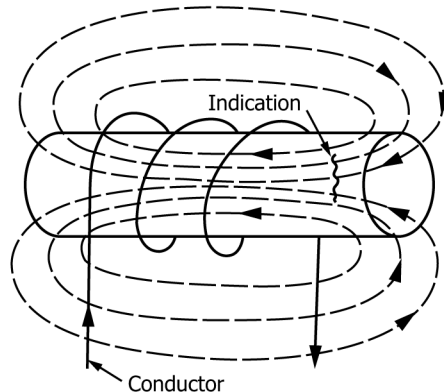
FIG. 1 Longitudinal Magnetization
