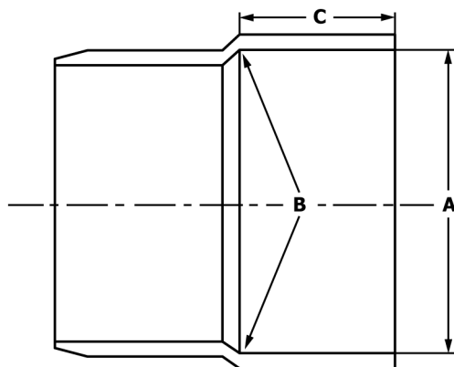
FIG. 2 Socket Dimensions
