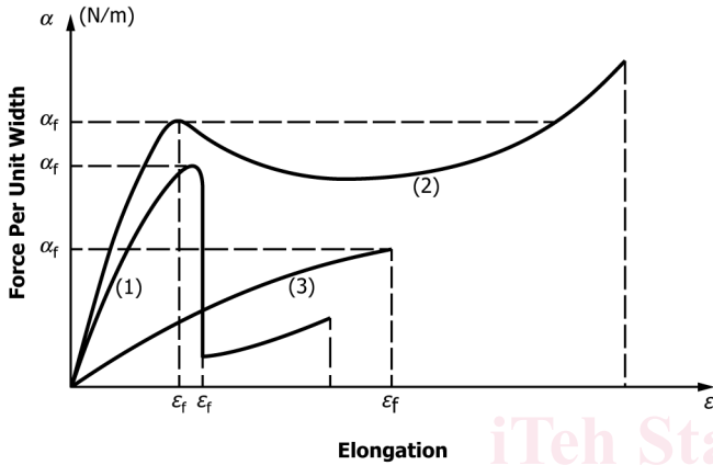
FIG. X1.1 Geomembrane Failure Patterns
