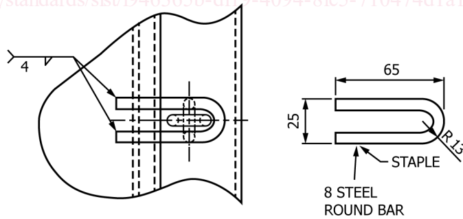
FIG. 3 Hasp
