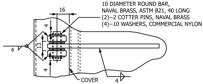
FIG. 2 Hinge
