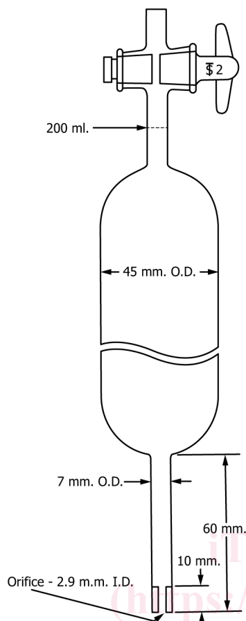
FIG. 1 Foam Pipet
