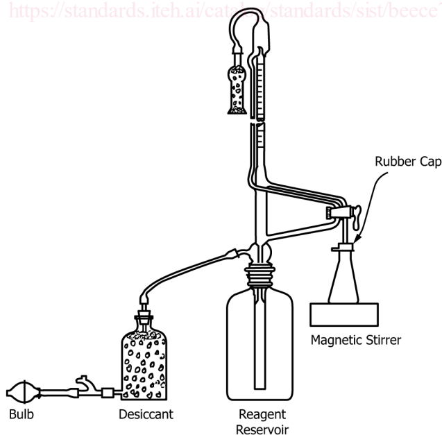
FIG. X1.1 Karl Fischer Titration Apparatus Assembly
