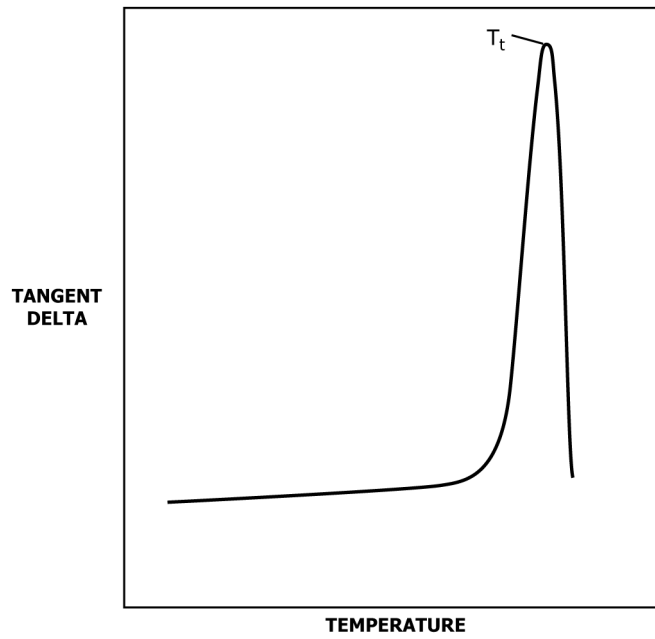
FIG. 3 Tangent Delta
