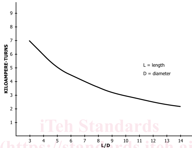
FIG. 7 Longitudinal Magnetization
