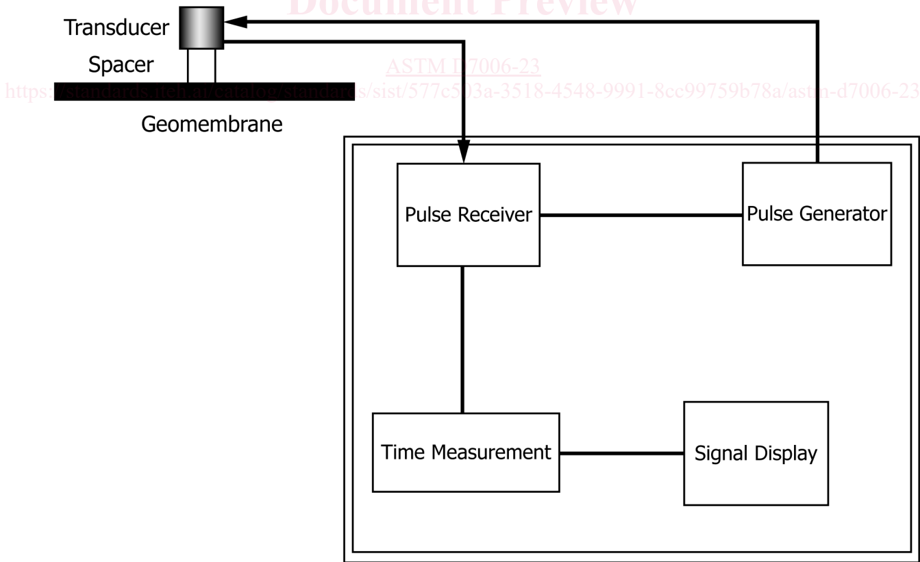
FIG. 1 Test Apparatus
