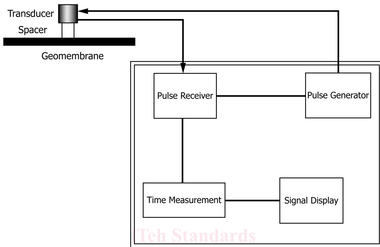
FIG. 1 Test Apparatus
