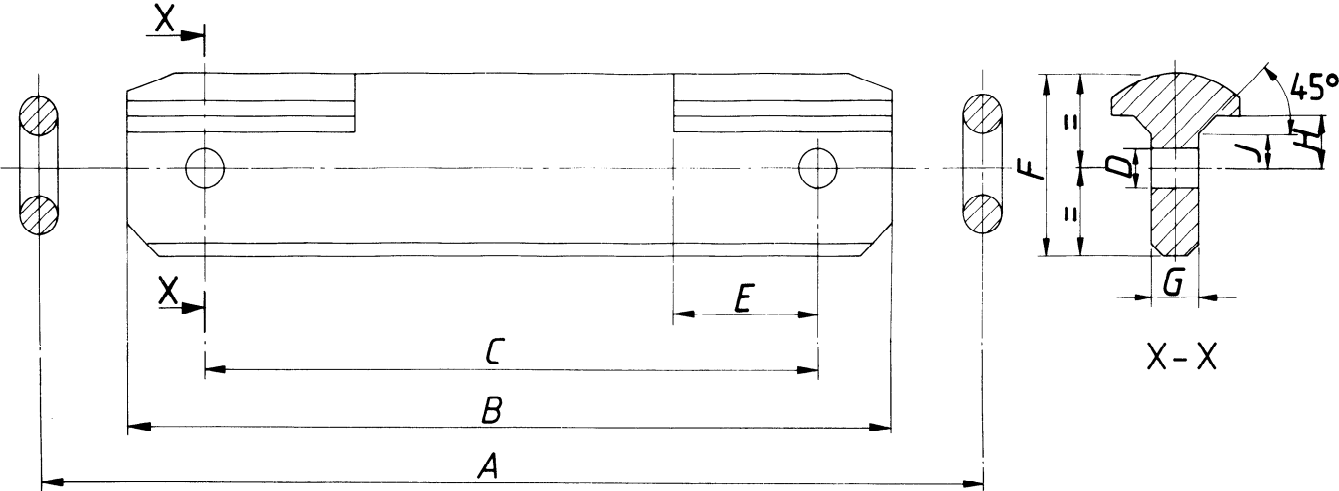
iTeh STANDARD PREVIEW Figure 1 — Dimensions des raclettes en T (standards.iteh.ai)
