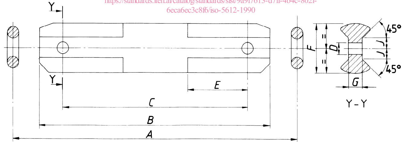
Figure 2 — Dimensions des raclettes en I
