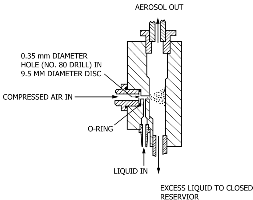
FIG. 2 Atomizer
