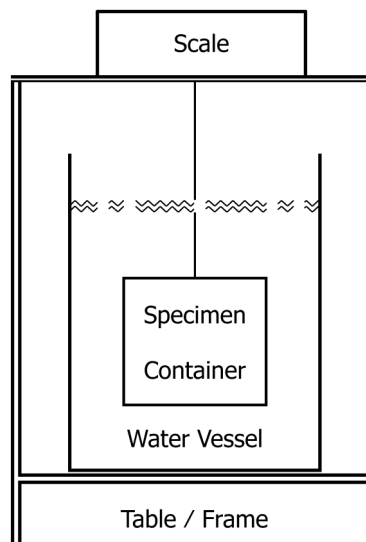
FIG. 1 Example Apparatus
