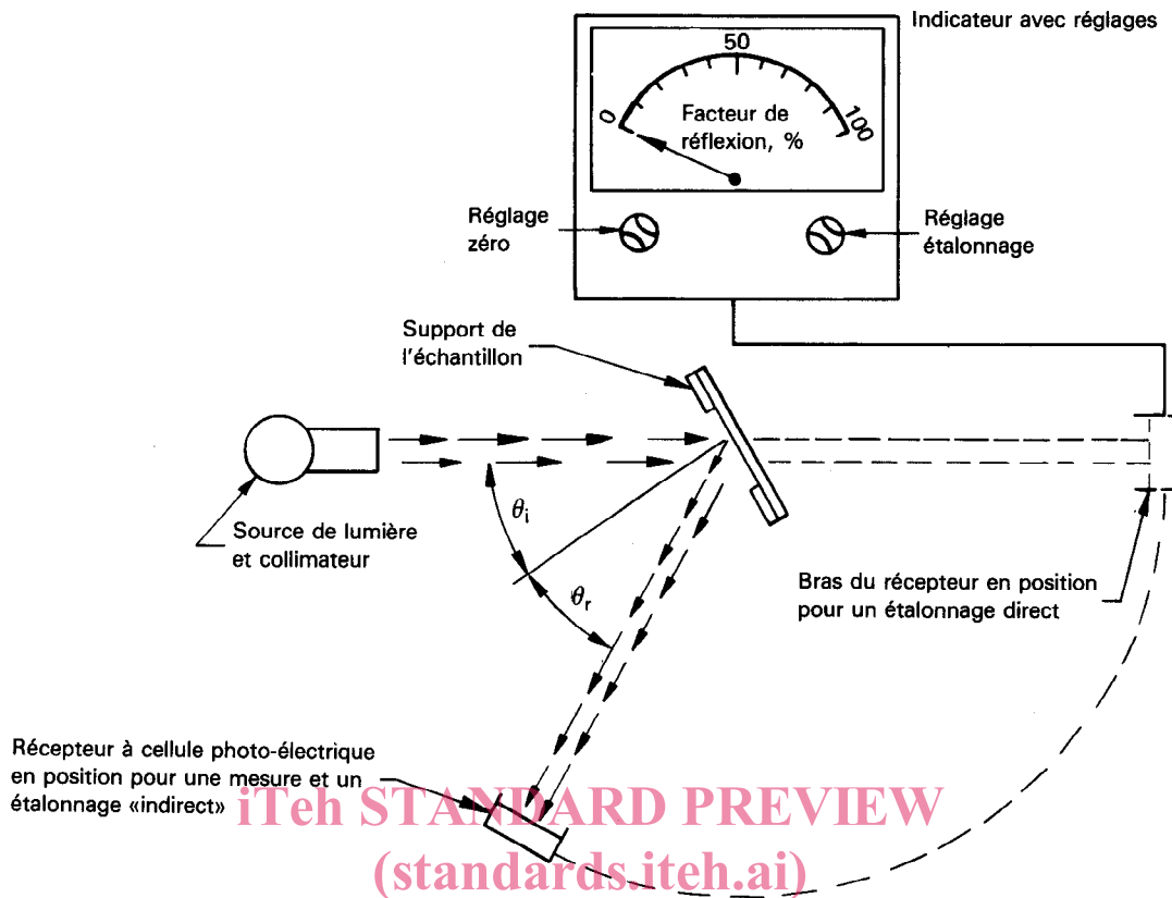
Figure 1 — Schéma général du réflectomètre pour les deux méthodes d'étalonnage.
