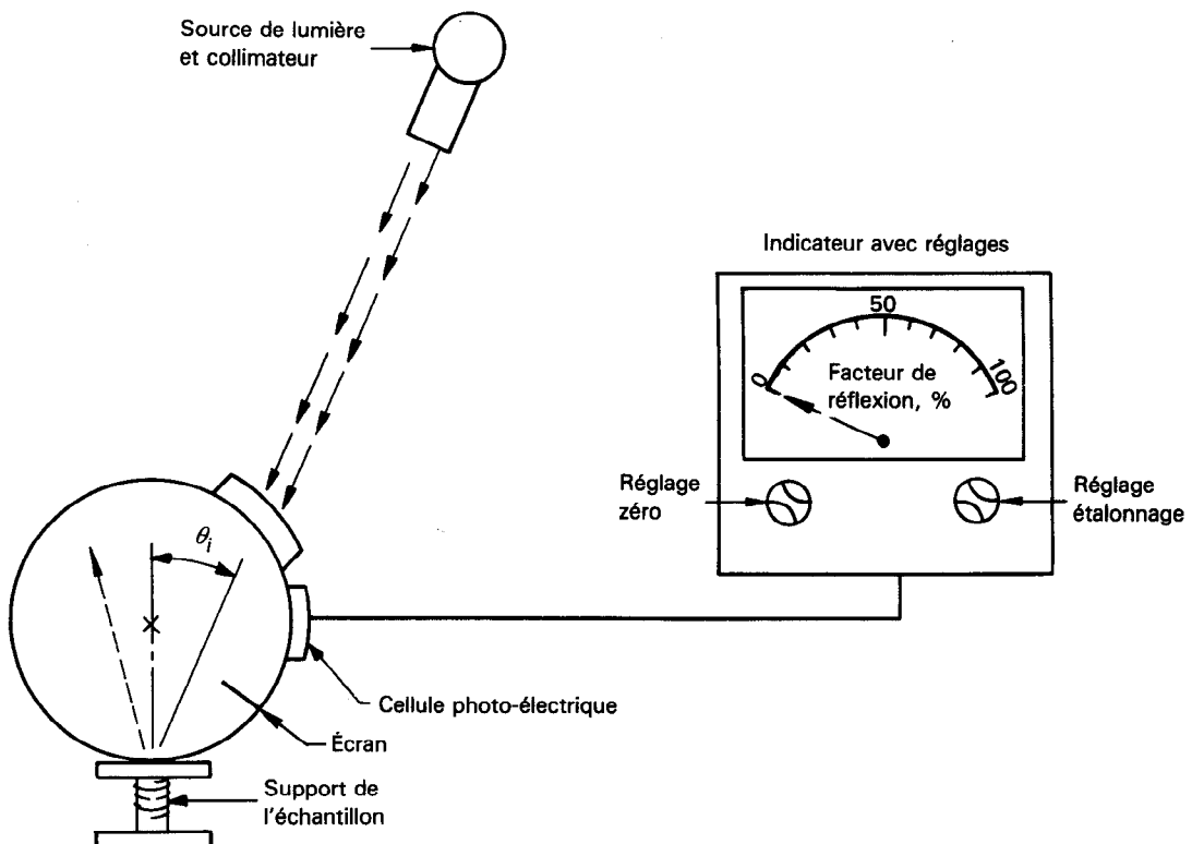
Figure 2 — Schéma général du réflectomètre dont le récepteur comprend une sphère d'Ulbricht.
