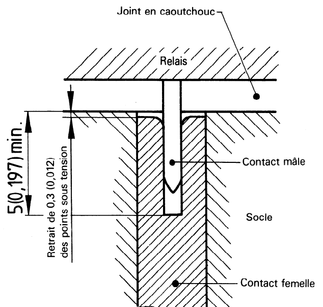
Figure 6 – Dimensions du contact femelle
