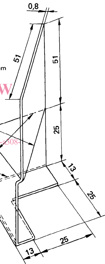
b) Moulage en équerre (extérieur)
