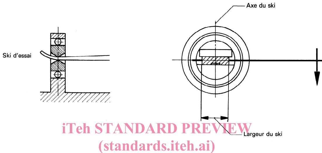
Figure 3 — Dispositif d'application de la charge pour l'essai de torsion des skis alpins
