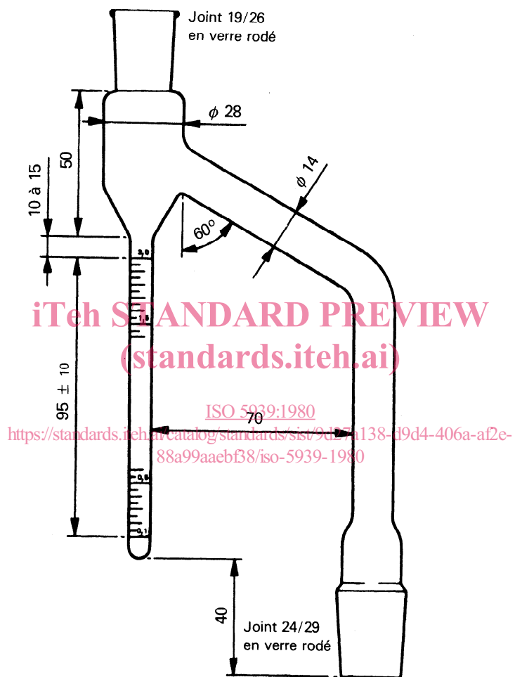
Figure 3 — Tube de recette de 2 ml (5.1.2)
