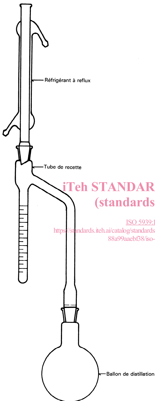
Figure 1 — Ensemble type de l'appareil de Dean et Stark (5.1)
