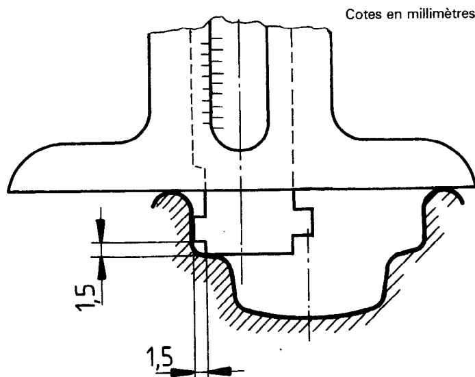
Figure B.5 — Calibre à vernier (graduations de 1/20 mm)
