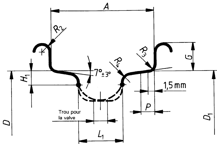
Figure 1 — Profil des jantes à repos de talon du pneu incliné (rebord droit)
