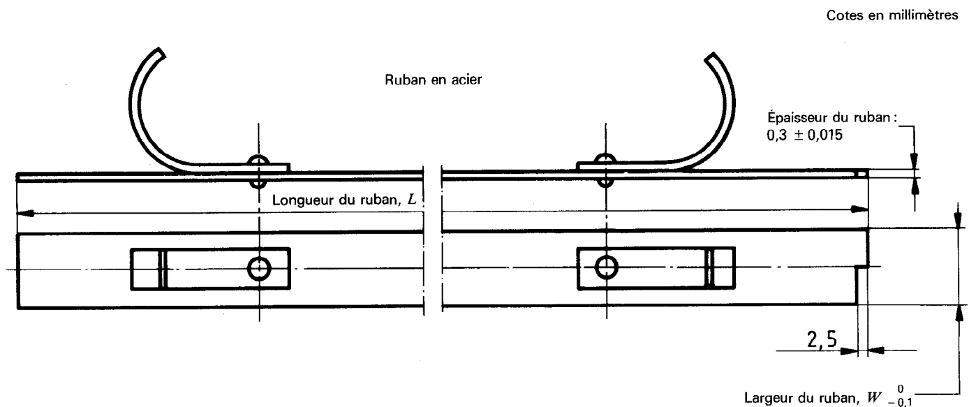
Figure B.3 — Détails du ruban
