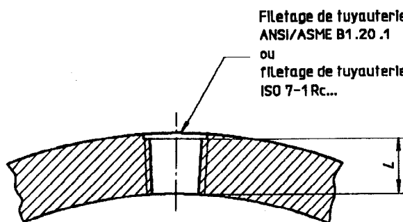
Figure 4 — Longueur de filetage des raccords auxiliaires
