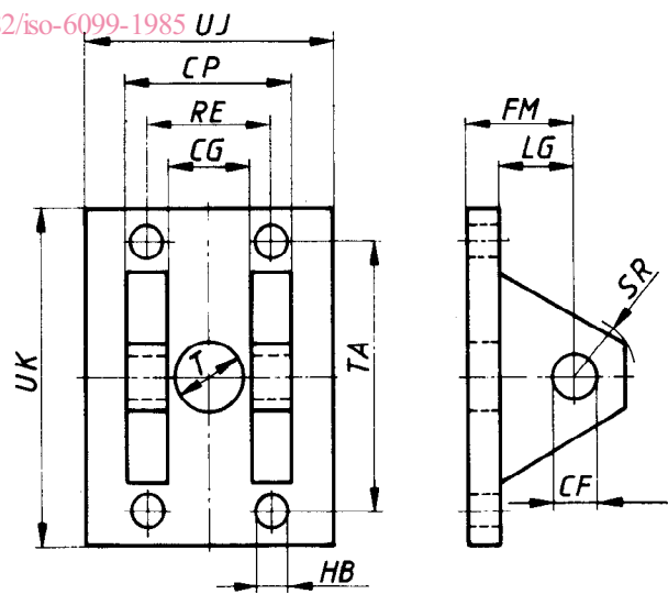
f) Chape rapportée pour rotule
