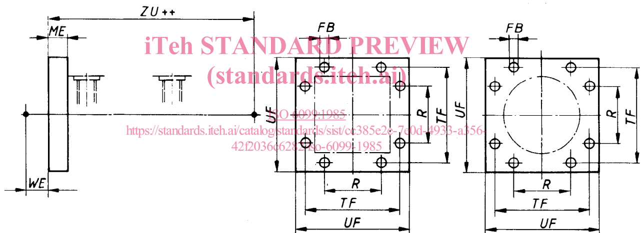
Figure 20 — (MDF 5) Bride avant carrée — Vérin double tige
