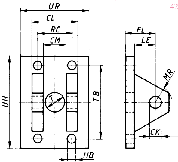
e) Chape rapportée
