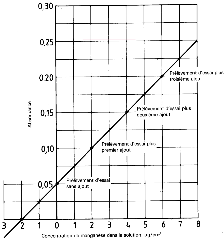
Figure A.1 — Exemple de courbe obtenue en utilisant la méthode des ajouts dosés
