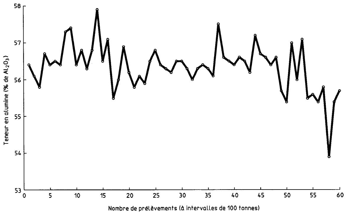
Figure 2 — Teneur en \text{Al}_2\text{O}_3 des différents prélèvements effectués dans un lot de minerai alumineux à intervalles de 100 tonnes
