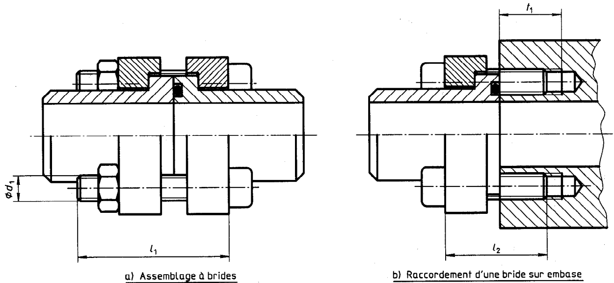
Figure 1 — Assemblage à brides et raccordement d'une bride sur embase — Pressions d'utilisation 25 MPa et 40 MPa (250 bar et 400 bar) (voir tableaux 1 et 2)
