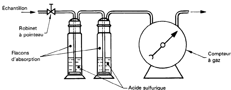
Figure — Appareil d'absorption
