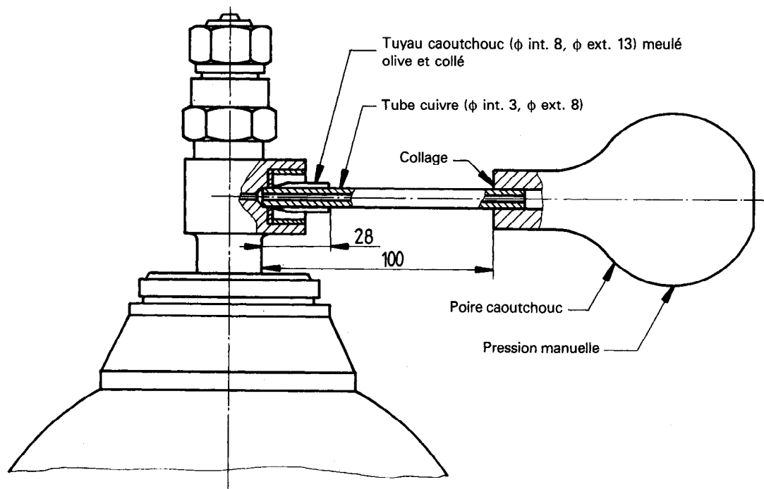
Figure B.1 — Dispositif permettant de détecter l'obstruction du robinet d'une bouteille à gaz
