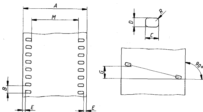
Figure B.1 — Dimensions des perforations pour les papiers en rouleaux utilisés dans les appareils de photocomposition et de phototirage
