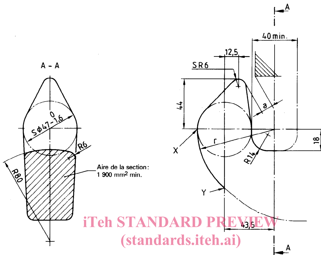
ISO 6489-1:1991 Figure 1 — Dimensions du crochet https://standards.iteh.ai/catalog/standards/sis/6765501c-18c5-4e89-9169-ecfd0d4e4cc4/iso-6489-1-1991
