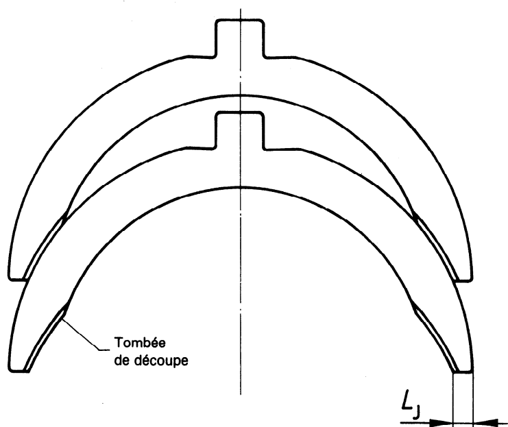
Figure 2 — Tombée de découpe des flasques à découpe imbriquée
