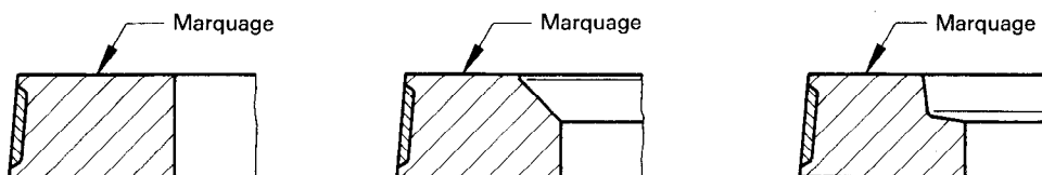
Figure 15 — Segments du type M incrustés
