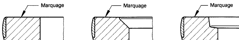
Figure 10 – Segments du type B semi-incrustés
