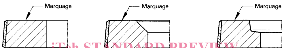
Figure 13 — Segments du type M à portée totale
