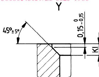
Figure 6 – Arêtes intérieures chanfreinées
