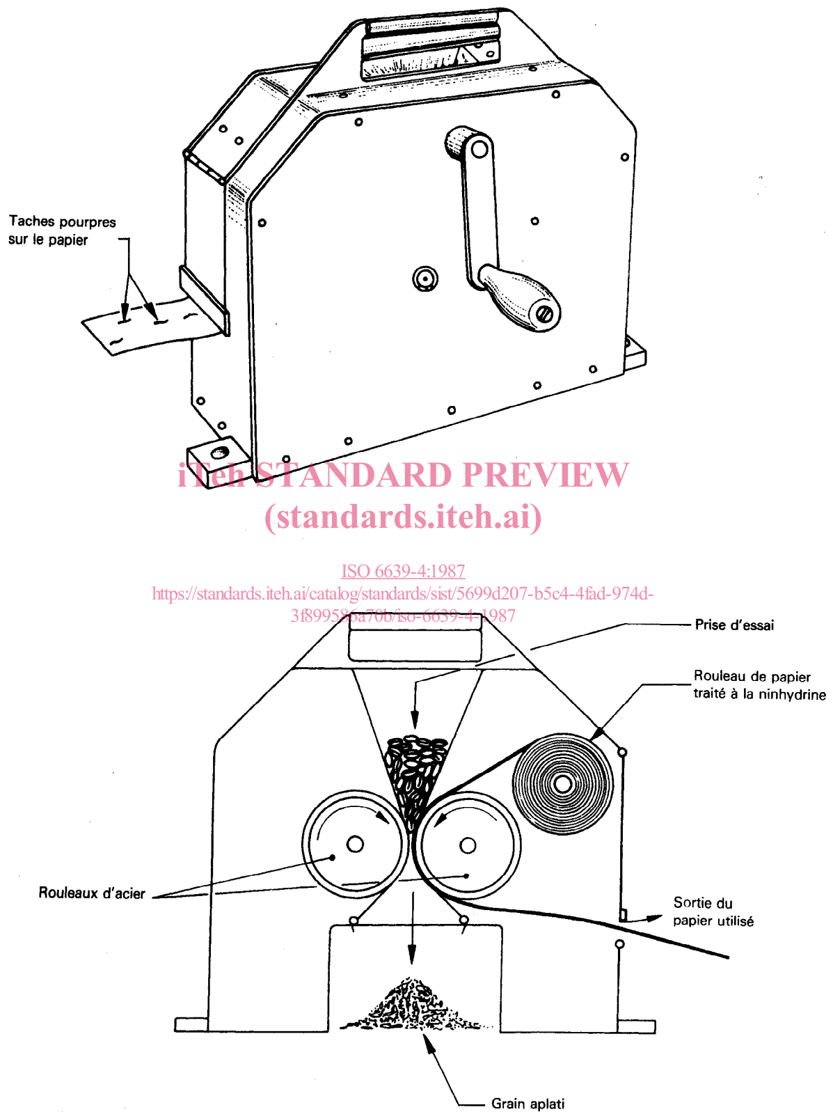
Figure 3 — Exemple d'appareil pour la détection de l'infestation cachée par le papier à la ninhydrine
