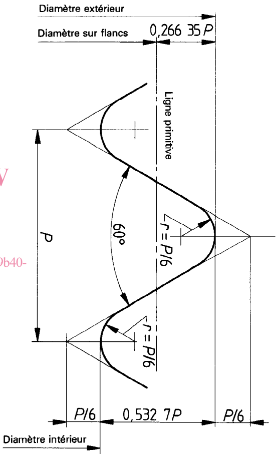
a) Profil de base du filetage BSC
