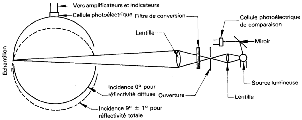
Figure 1 – Plan optique schématique d'un réflectomètre à sphère pivotante
