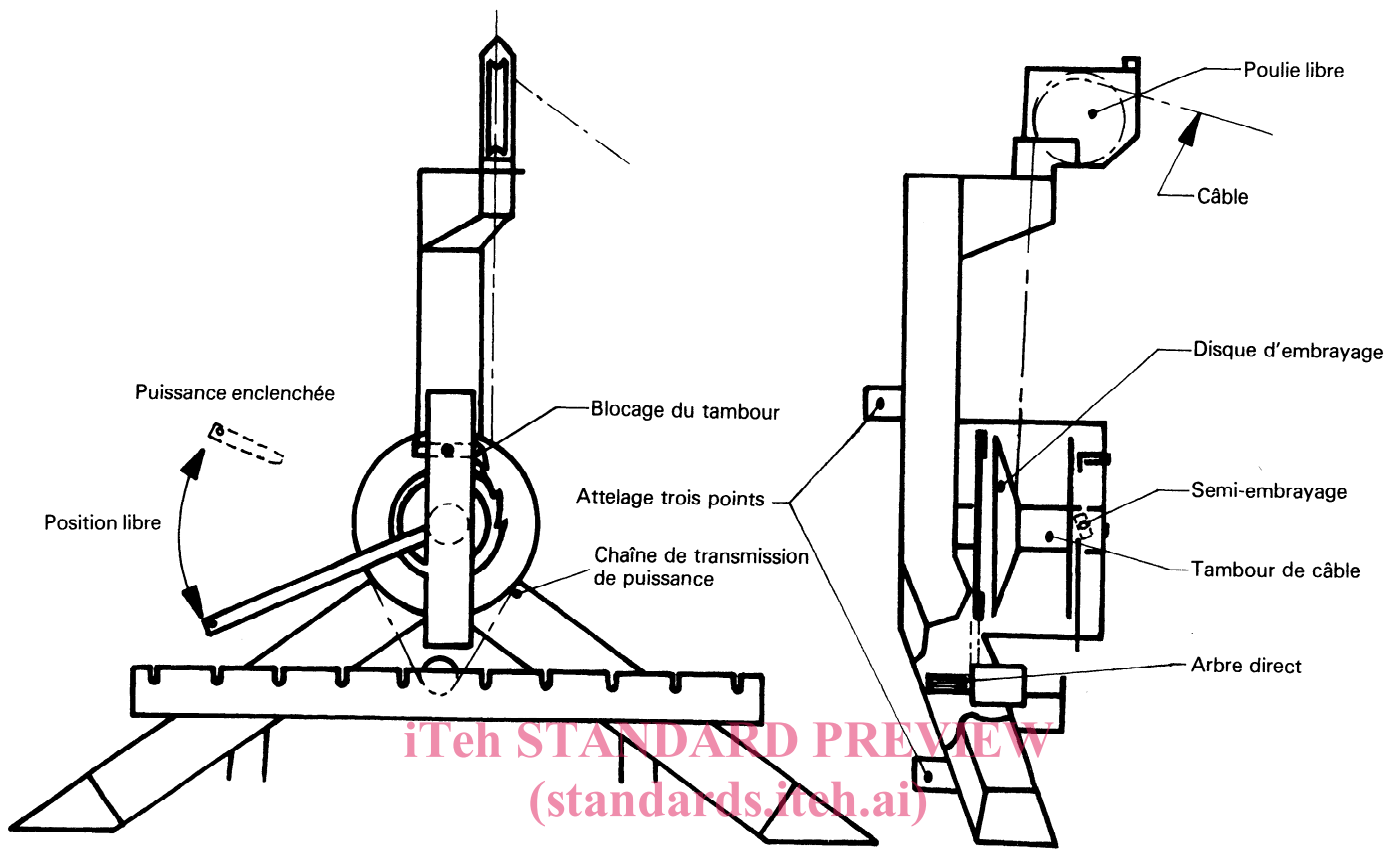
ISO 6816:1984 https://standards.iteh.ai/standards/iso-6816-1984/iso-6816-1984-43815244988f/iso-6816-1984 Figure 3 — Treuil sur attelage trois points
