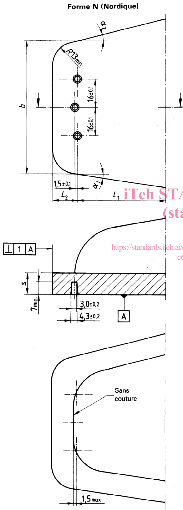
Figure 1 — Partie avant de la chaussure de forme N (Nordique)
