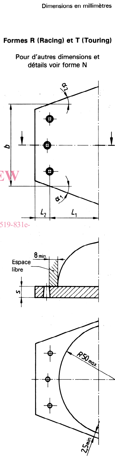
Figure 2 — Partie avant de la chaussure de formes R (Racing) et T (Touring)
