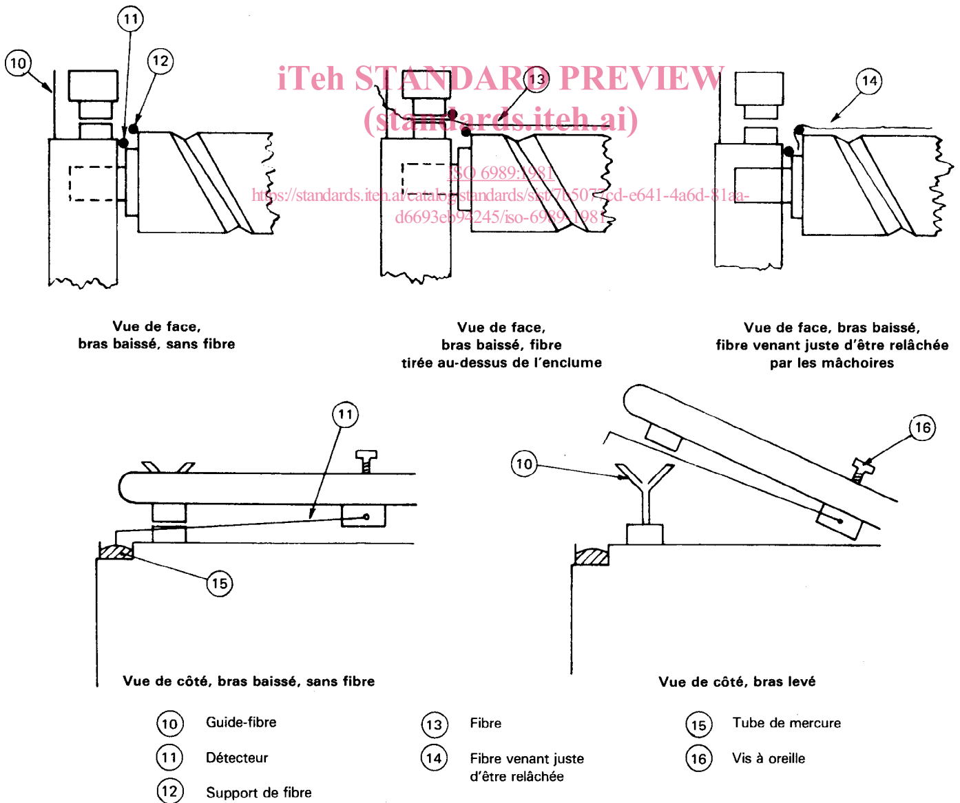
Figure 2 – Détails de l'appareil
