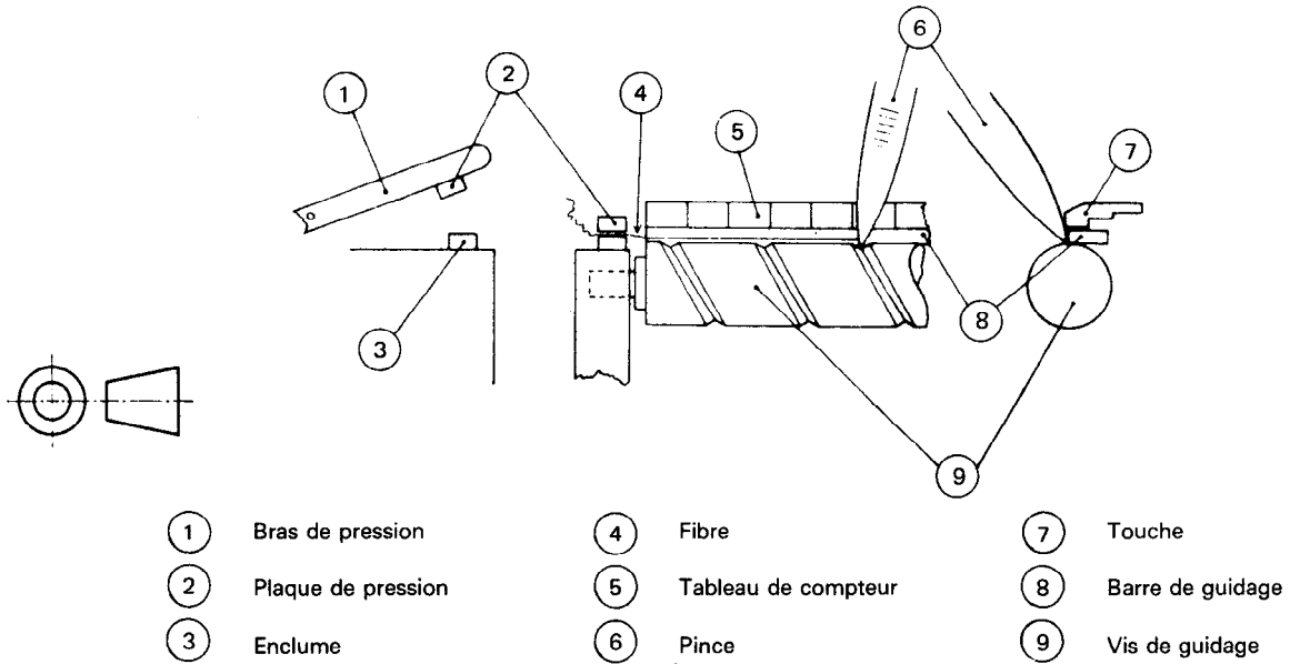
Figure 1 – Parties essentielles de l'appareil pour le mesurage de la longueur des fibres individuelles – Détecteur non visible
