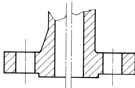
Type 21 Bride incorporée à un appareil
