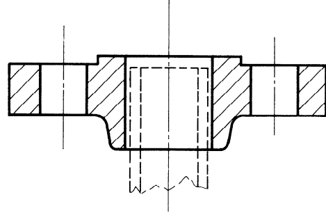
Type 12 Bride à emmancher à souder à collerette
