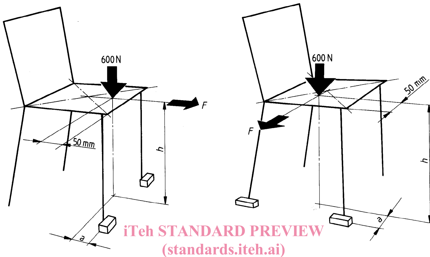
ISO 7174-1:1988 Figure 1 — Basculement avant et basculement latéral pour les chaises sans accotoirs https://standards.itech.ai/catalog/standards/sist/8294-decf-09a7-41b9-8c00-52ab9f147d33/iso-7174-1-1988
