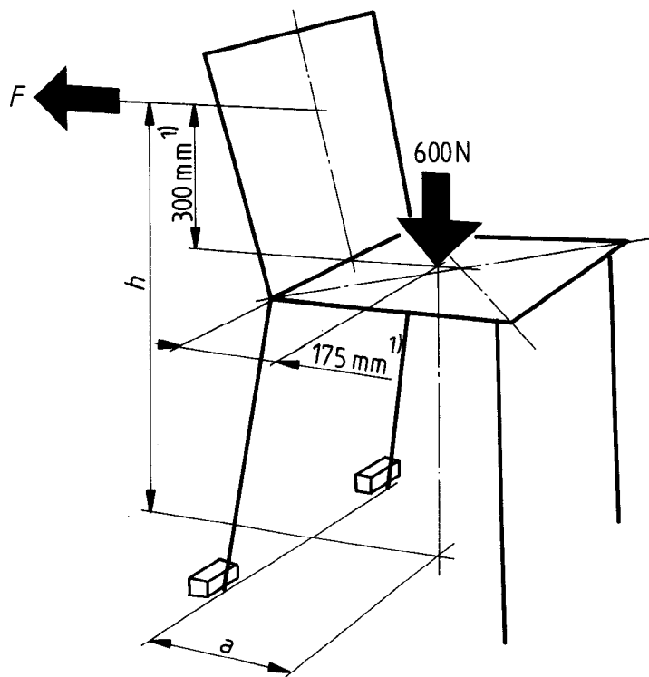
ISO 7174-1:1988 Figure 1 — Basculement avant et basculement latéral pour les chaises sans accotoirs https://standards.itech.ai/catalog/standards/sist/8294-decf-09a7-41b9-8c00-52ab9f147d33/iso-7174-1-1988
