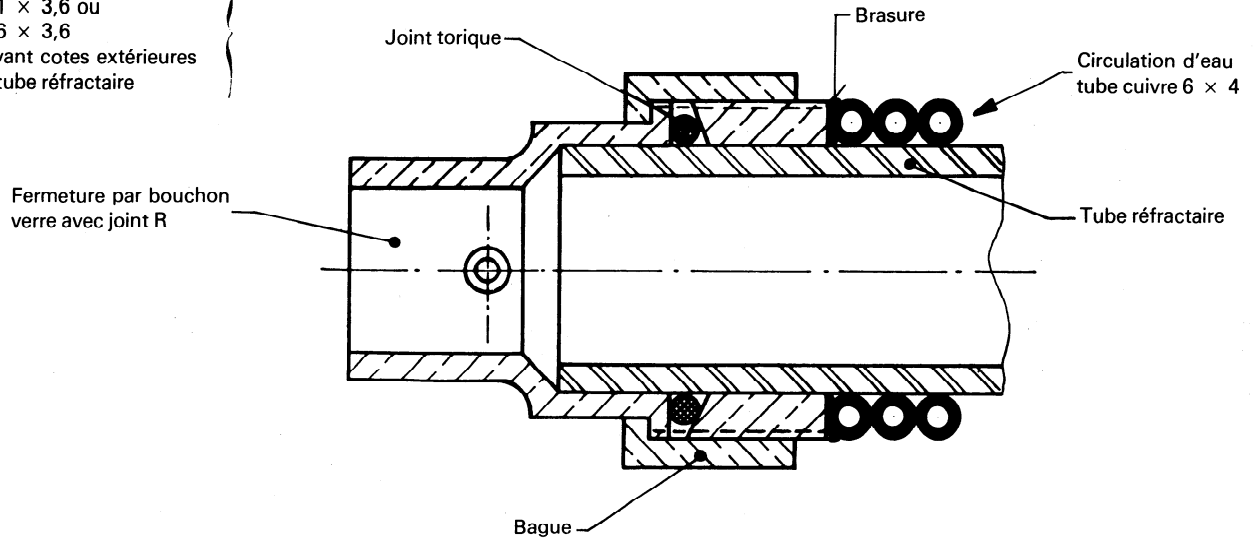
Figure 3 — Tête métallique réfrigérée pour tube à combustion
