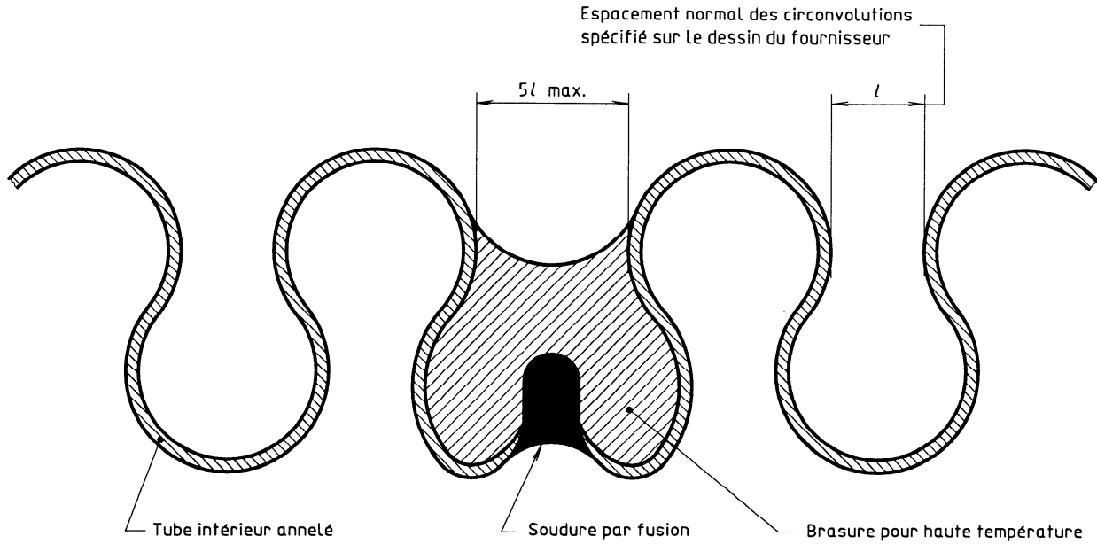
Figure 1 — Configuration du raboutage du tube intérieur
