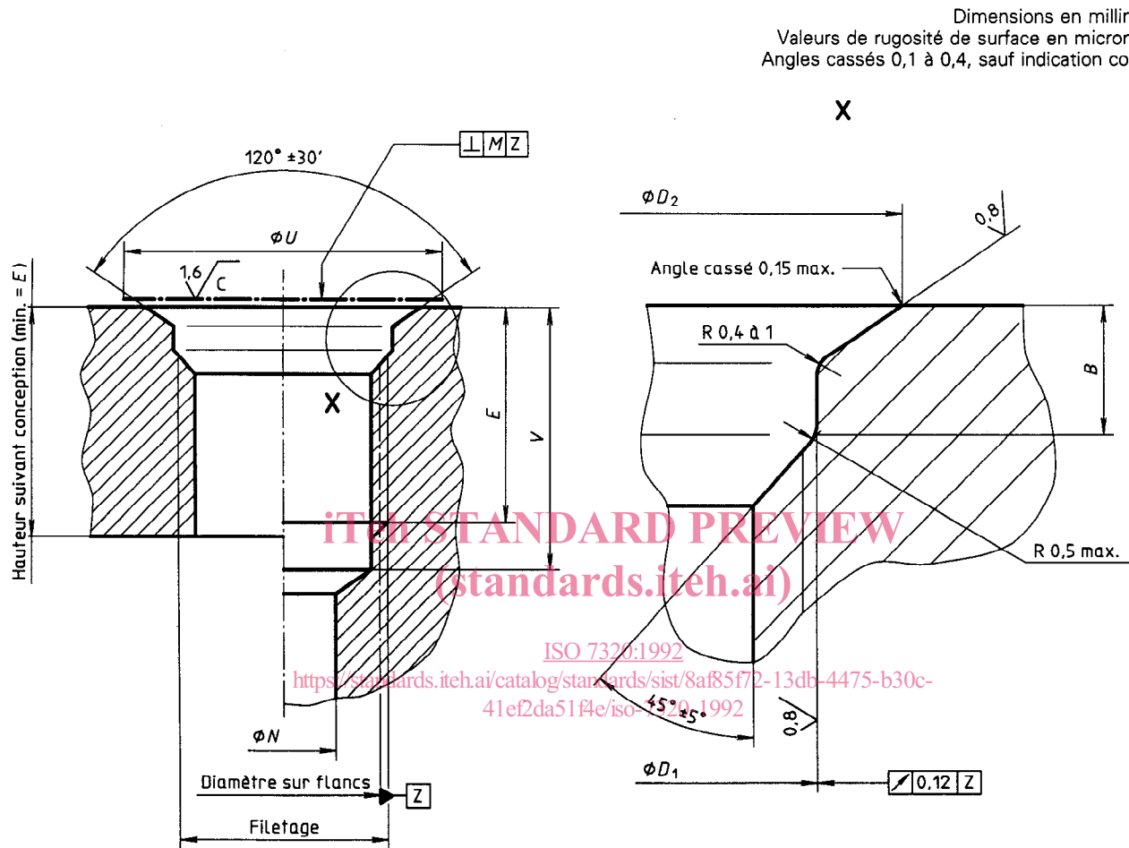
Figure 1 — Configuration de l'orifice de raccordement fileté
