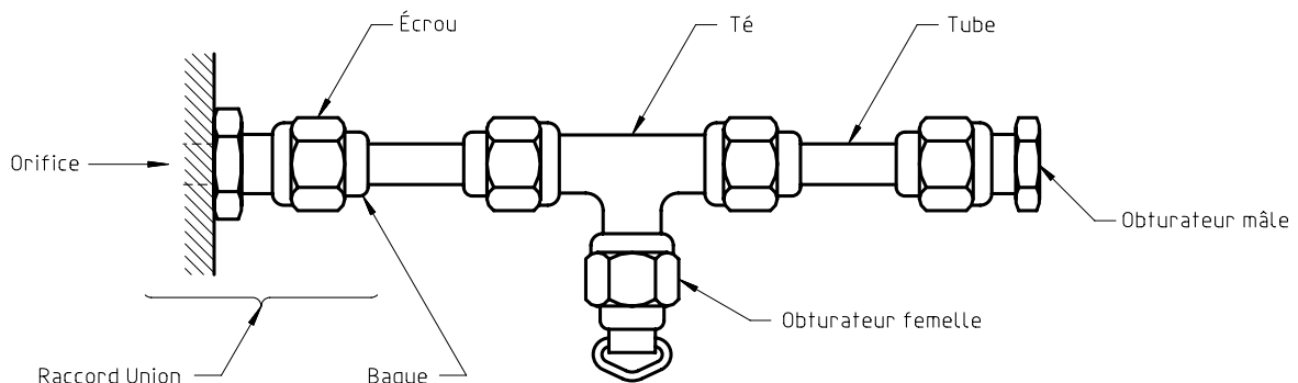
Figure 1 — Désignation des éléments de raccordement
