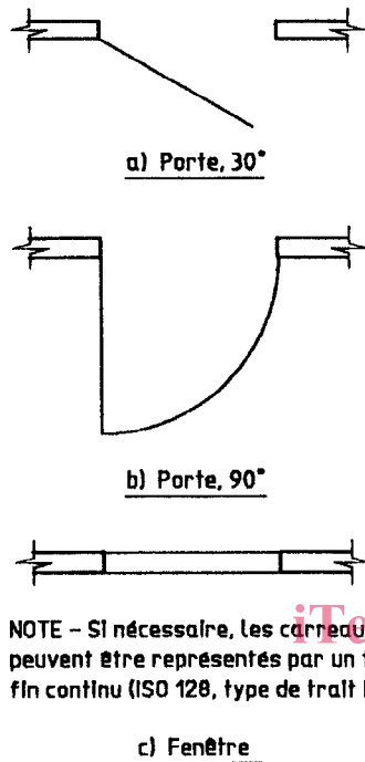
Figure 7 — Exemples de portes et fenêtres sur des dessins à petites échelles
