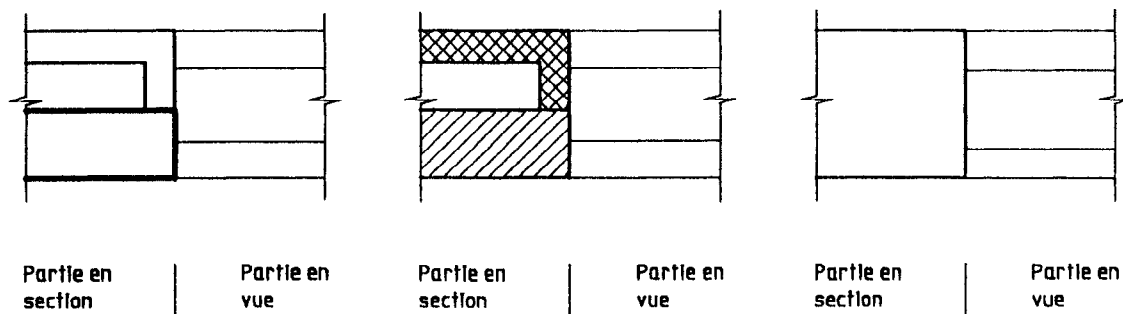
Figure 1 — Exemples de contours des parties en section et en vue
