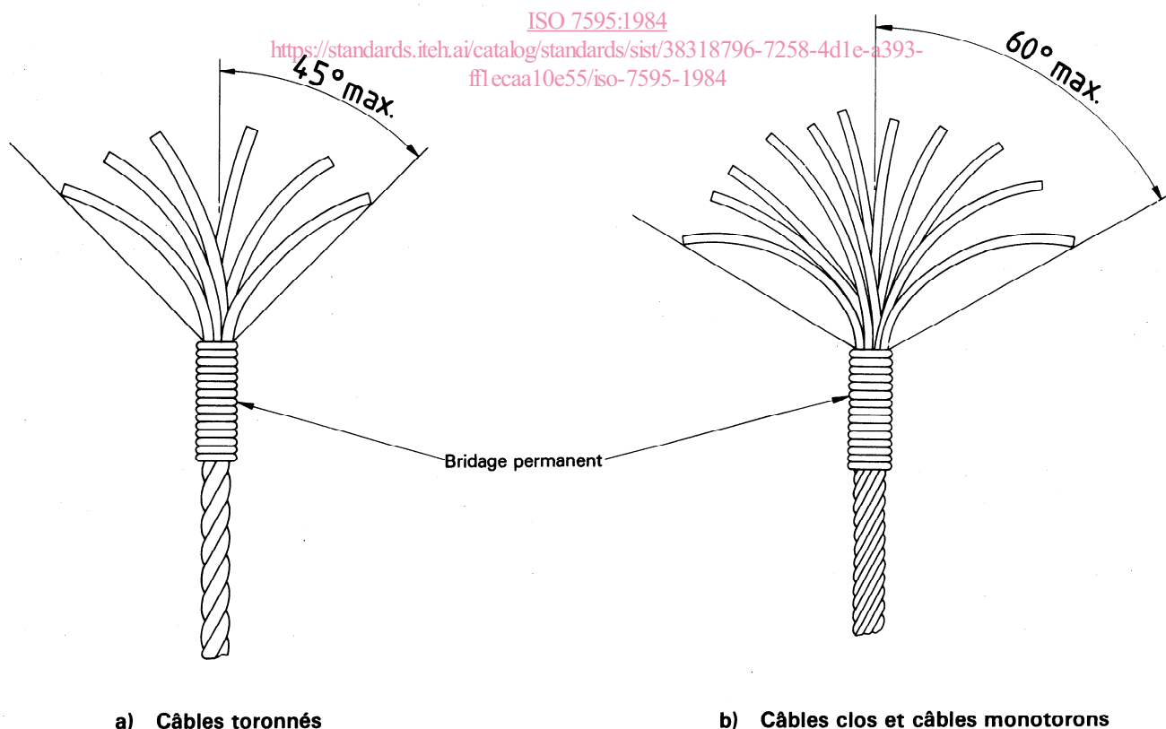
Figure — Angle d'ouverture du faisceau
