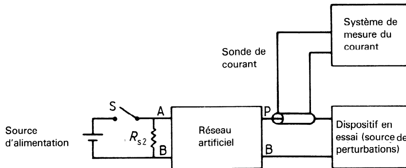
Figure 2 – Montage d'essai pour le mesurage des transitoires de courant
